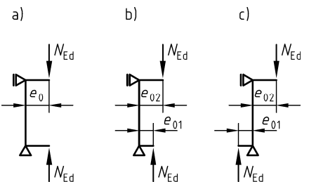
(DIN 1045-1, Bild 13)
