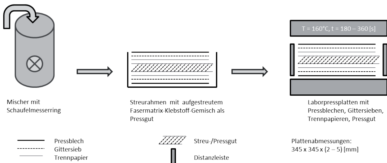
Abb. 2: Verfahrensschema der Herstellung der düBraFa im Labormaßstab
