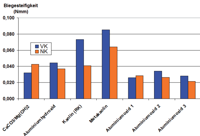
Abb. 5: Biegesteifigkeit (VK: vor Kalander, NK: nach Kalander)
