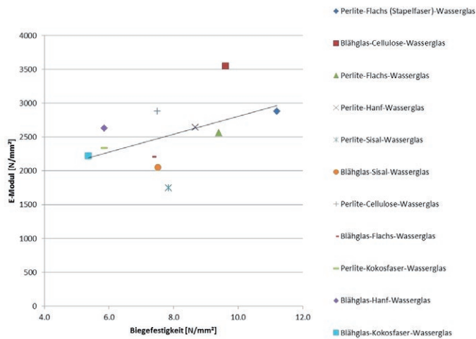
Abb. 3: Korrelation der ermittelten Biegefestigkeit und des E-Moduls in Abhängigkeit der verwendeten Rohstoffvariante
