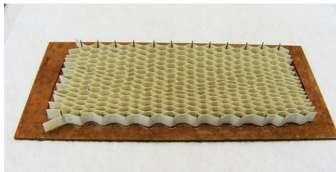
Abb. 7: Manuelle Herstellung von Expansionswaben mit mineralisch hochgefüllten auf der Technikumpapiermaschine hergestellten Papieren
