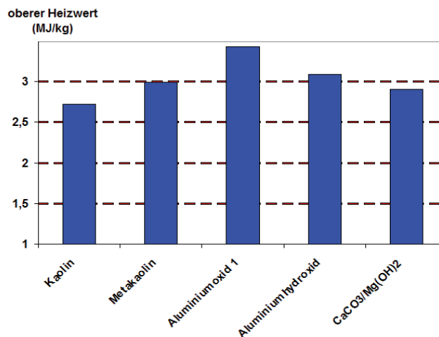
Abb. 6: Heizwert (Laborblätter ohne Mineralfaserzusatz)
