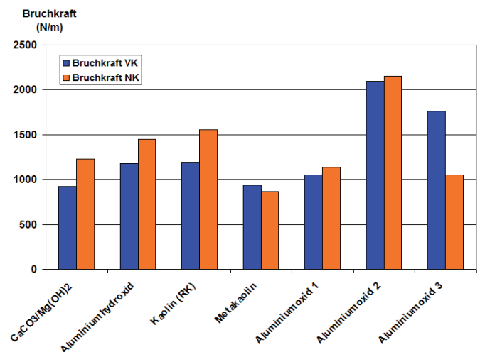
Abb. 4: Breitenbezogene Bruchkraft (VK: vor Kalandern, NK: nach Kalandern)
