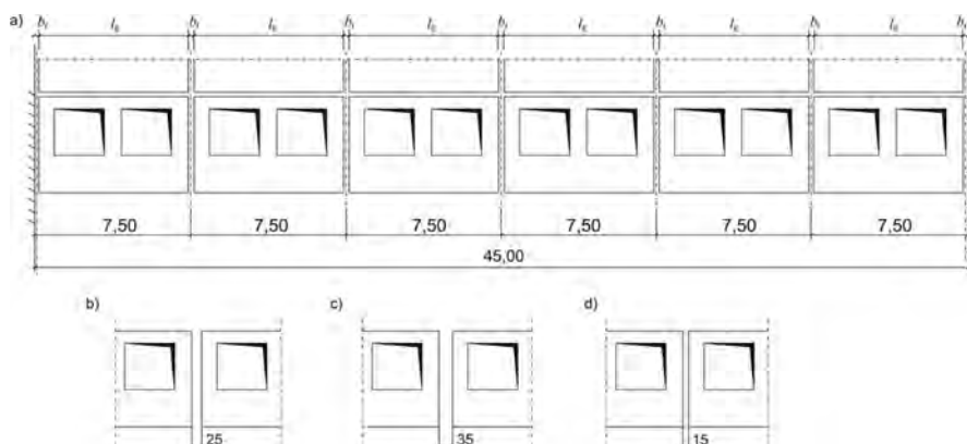
Abb. 2.6 Fugenbreiten bei vorherigem Aufmaß; a) Ansicht und Abmessungen der Fassade, b) Nennmaß der Fugenbreite, c) maximale Fugenbreite, d) minimale Fugenbreite.
